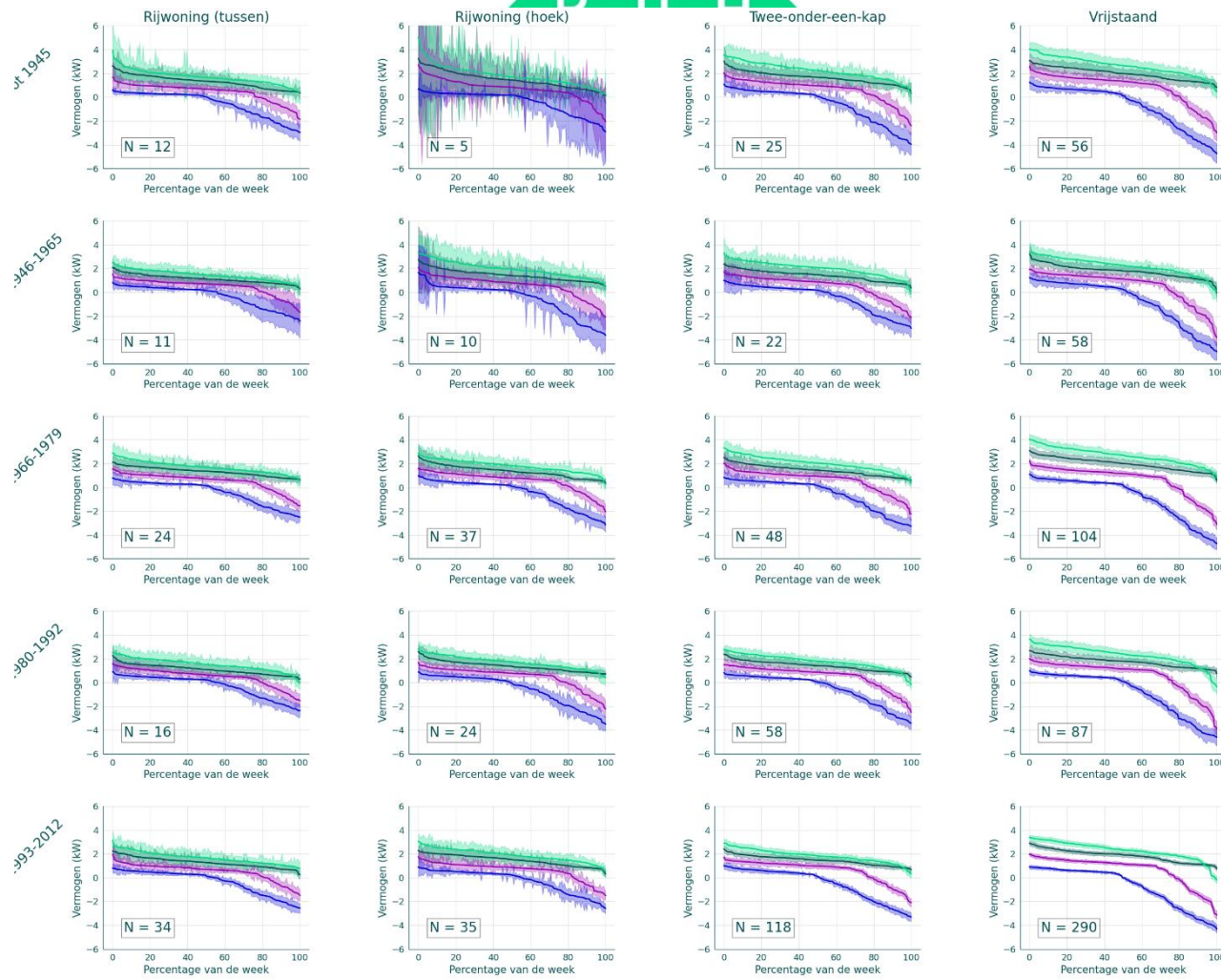
Figuur C.3 Belastingduurkromme van all-electric warmtepompen over vier referentieweeken (woningtype, bouwperiode)
