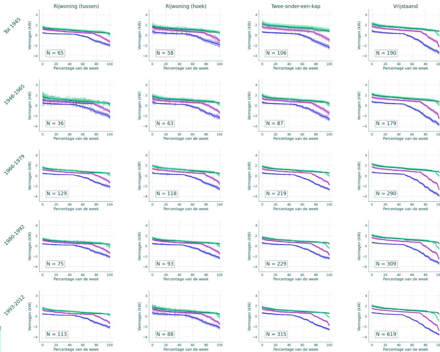
Figuur B.3 Belastingduurkromme referentieweek woningen met hybride warmtepomp (clusters: bouwperiode, woningtype)
