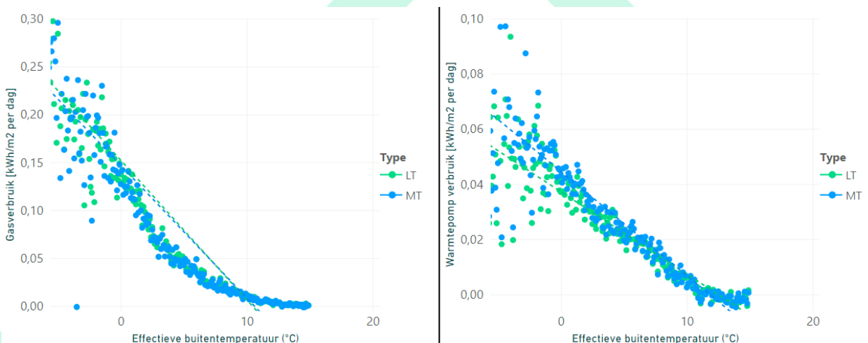
Figuur 4 - Invloed van afgiftetemperatuur in de woning op gasvraag (links) en elektriciteitsvraag (rechts) van hybride warmtepompen. Het gemiddelde energieverbruik in kWh/m² per dag is uitgezet tegen de effectieve buitentemperatuur.
