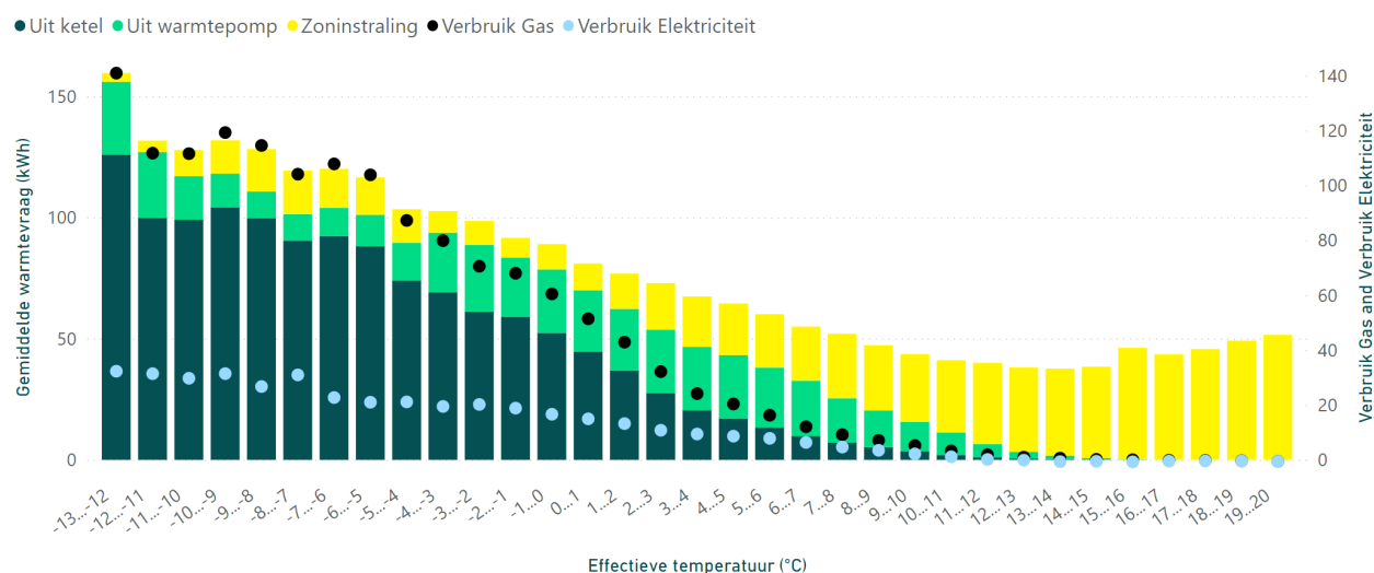
Figuur 17 - Invulling van de warmtevraag door de gasketel, warmtepomp en zoninstraling. Vooral bij temperaturen tussen 0 en 13 °C neemt de warmtepomp een groot deel van de invulling van de warmtevraag voor zijn rekening. Let op: voor zeer koude dagen lijkt de invulling van de warmtepomp hoger te worden. Dit is echter een statistische fluctuatie gezien dankzij de beperkte hoeveelheid data bij die temperaturen en heeft verder geen betekenis.
