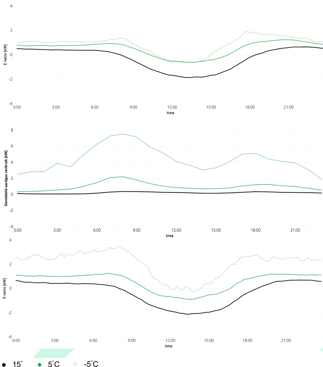
Figuur 20 - Gelijktijdigheid van hybride en all-electric warmtepompen. Boven het gemiddelde elektriciteitsgebruik van een hybride warmtepomp, in het midden het gemiddelde gasverbruik van dezelfde groep woningen en onder het gemiddelde voor all-electric warmtepompen. Voor alle grafieken geldt: zwart is bij 15°C, groen is bij 5°C en licht groen is bij -5°C effectieve temperatuur.
