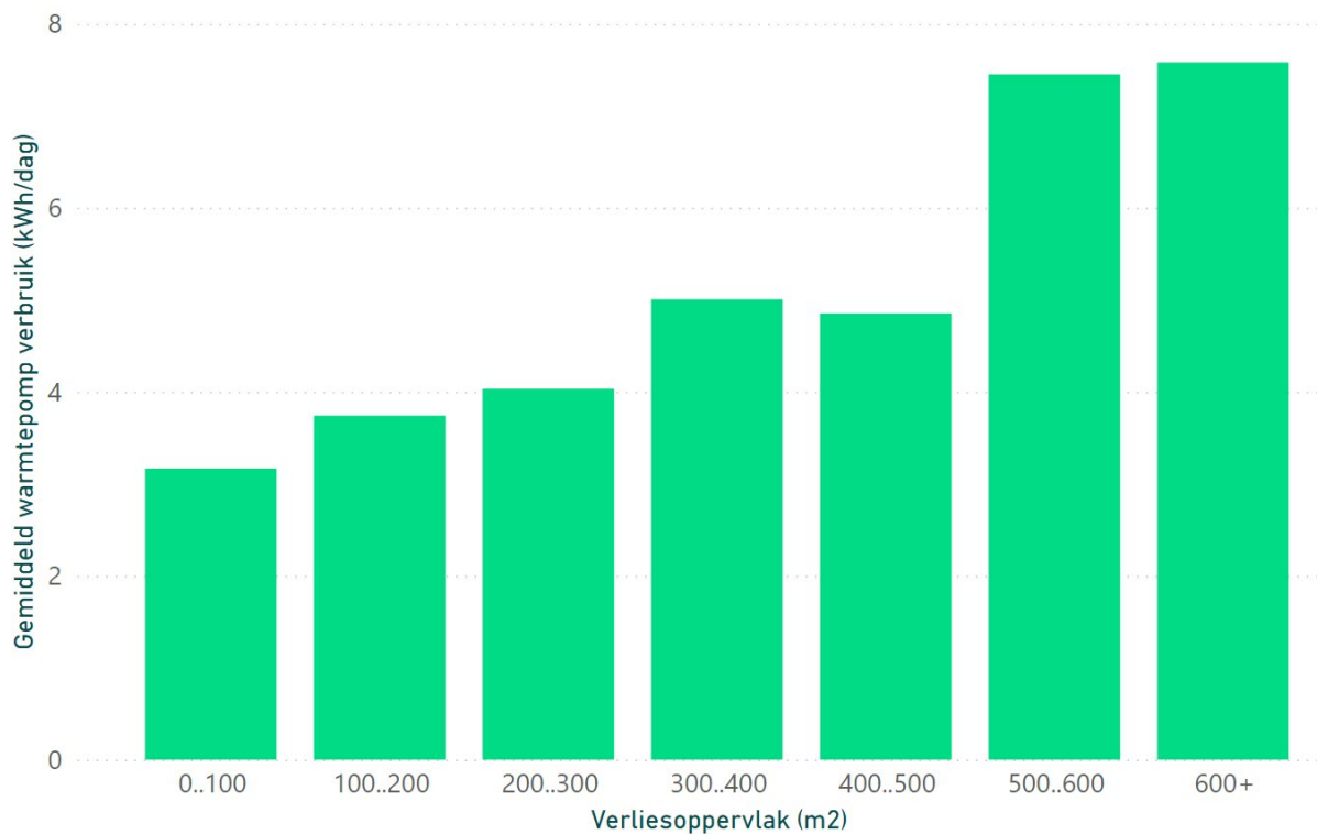
Figuur 5 - Het verliesoppervlak van de woningen in relatie tot het gemiddeld warmtepomp verbruik per dag (kWh).
