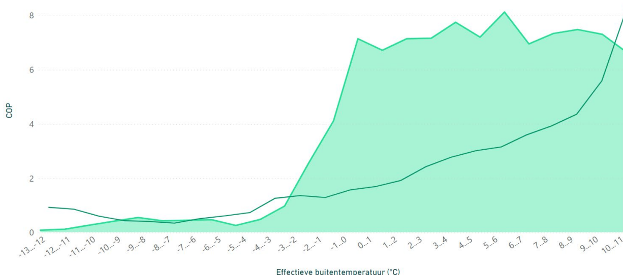
Figuur 19 - COP als functie van de effectieve buitentemperatuur. Op de achtergrond de frequentie waarmee de betreffende effectieve buitentemperatuur is voorgekomen in 2020-2021.
