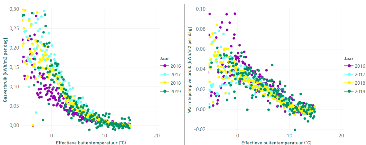
Figuur 1 – Gemiddeld energieverbruik in kWh/m 2 per dag (links gasverbruik en rechts elektriciteitsverbruik van de warmtepomp) in relatie tot de effectieve buitentemperatuur, uitgesplitst naar installatiejaar van de warmtepomp (hybride warmtepompen).
