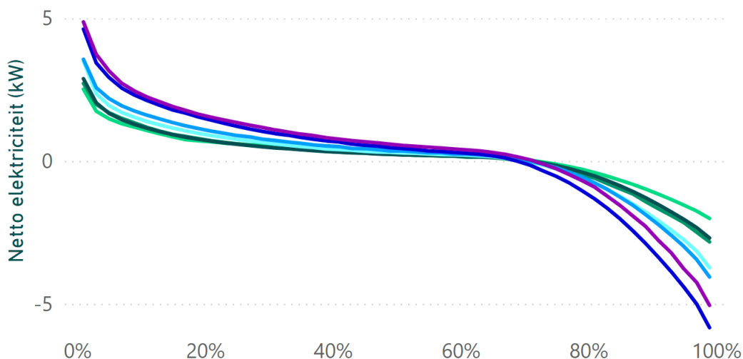
Figuur 13 - Belastingduurkromme voor hybride warmtepompen voor woningen met PV-panelen. De maximale afnamepiek schaaft met het verliesoppervlak per woning. Maximale afname en teruglevering zijn vergelijkbaar in vermogen.
