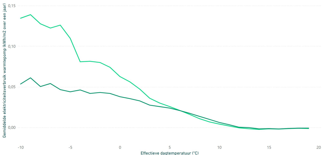
Figuur 21 - Gemiddeld elektriciteitsverbruik van de warmtepomp in kWh/m² per jaar uitgezet tegen de effectieve dagtemperatuur.
