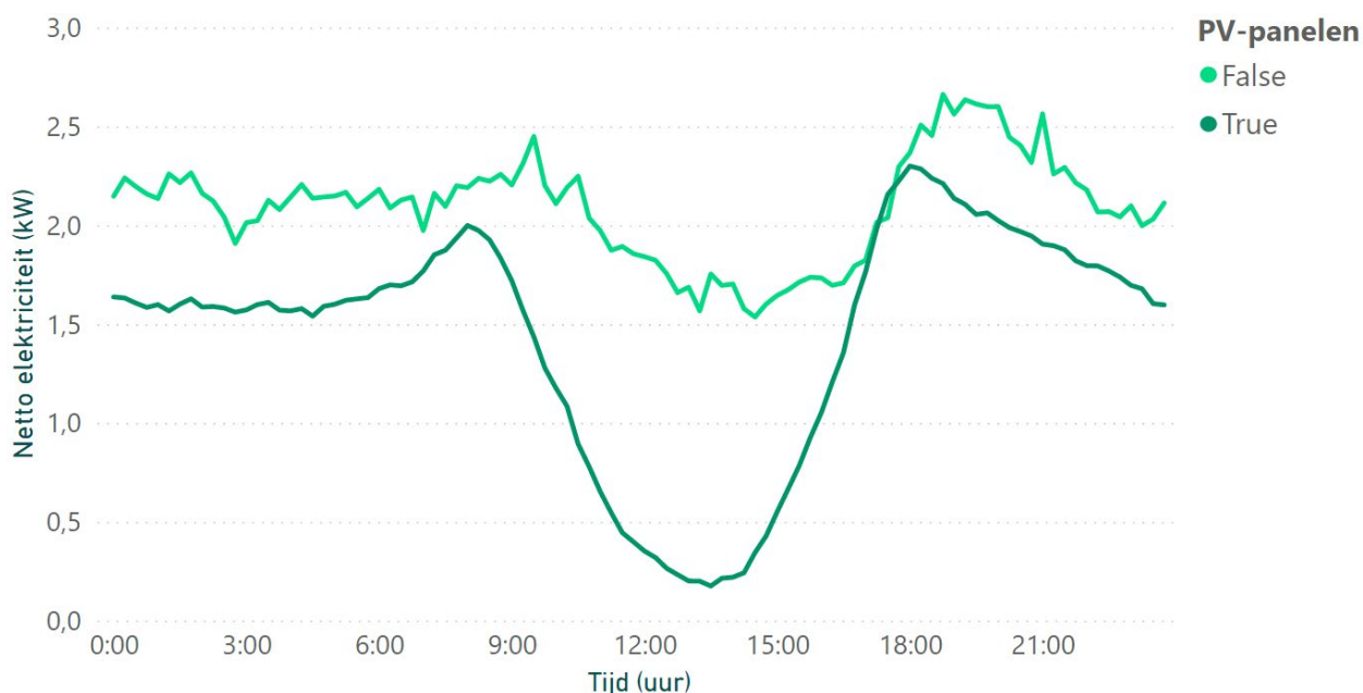
Figuur 12 - Vergelijking elektrisch profiel voor woningen met en zonder PV-panelen. Profiel gemiddeld voor alle warmtepompen over de vijf koudste dagen van de meetperiode.
