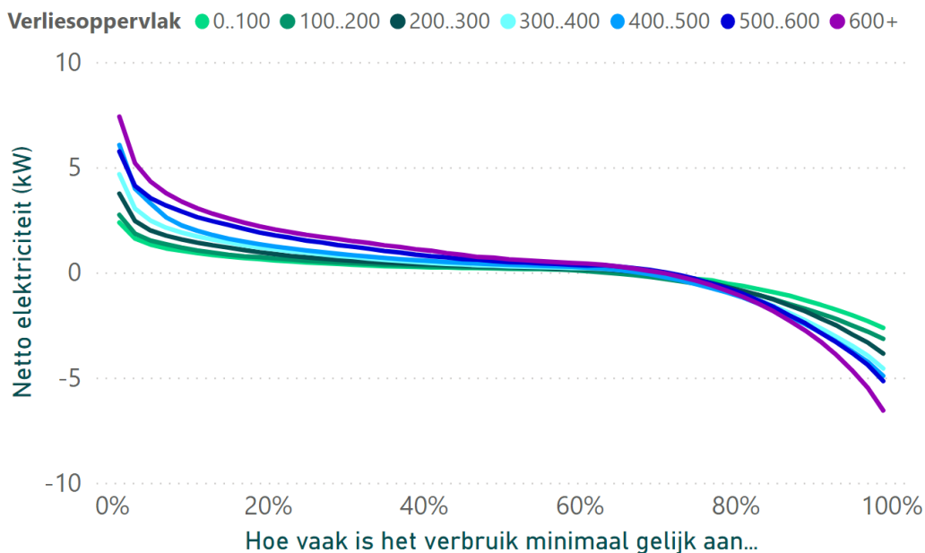
Figuur 15 - Belastingduurkromme voor all-electric warmtepompen, voor woningen mét PV-panelen. De terugleverpiek is qua omvang vergelijkbaar met de afnamepiek.
