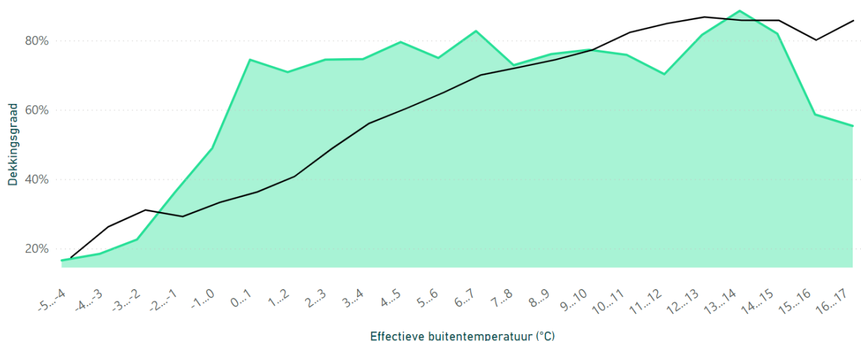
Figuur 18 - Dekkingsbijdrage van de warmtepomp uitgezet tegen de effectieve buitentemperatuur. De frequentie van iedere temperatuur is bekend (groene vlak). Hieruit volgt de totale dekking op jaarbasis.
